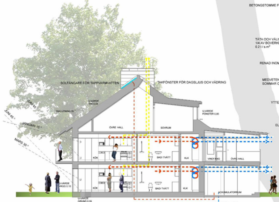
FUNKTIONSBILD
